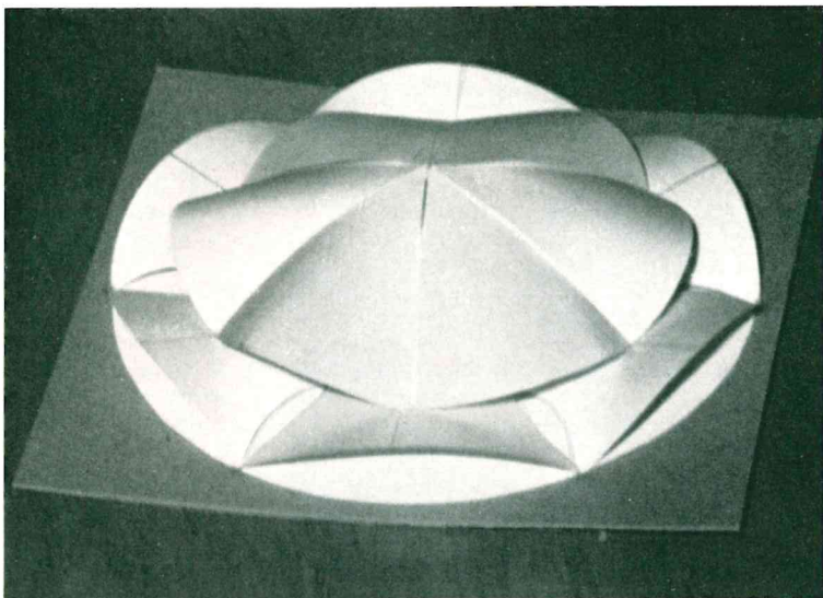
Im Kunstgeschichtsunterricht in UII wurde das Pantheon, die Hagia Sophia, die Palastkirche in Aachen als Beispiele von Zentralbauten besprochen. Das Bild zeigt das Modell eines modernen Zentralbaus. Zeichenpapier war so zu verformen und zusammenzusetzen, daß dadurch Steifheit des Materials entstand und eine große Fläche freitragend überwölbt werden konnte.
